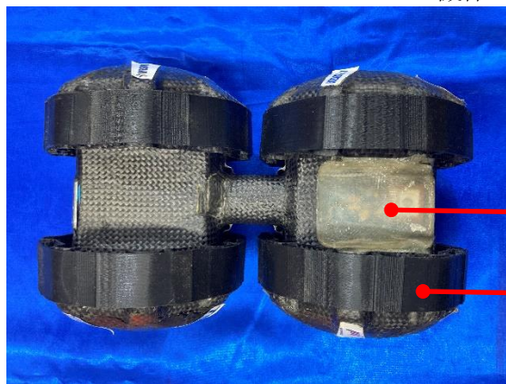
機体上面図
