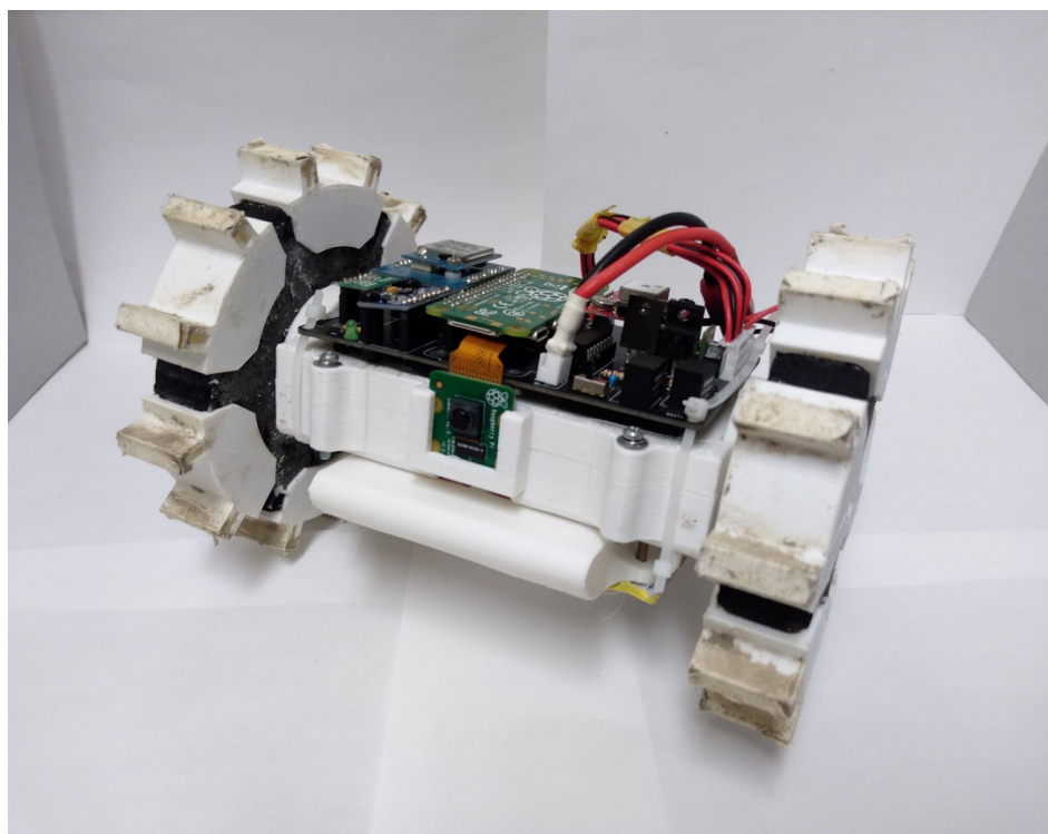
図4.1.3 実機外観図
