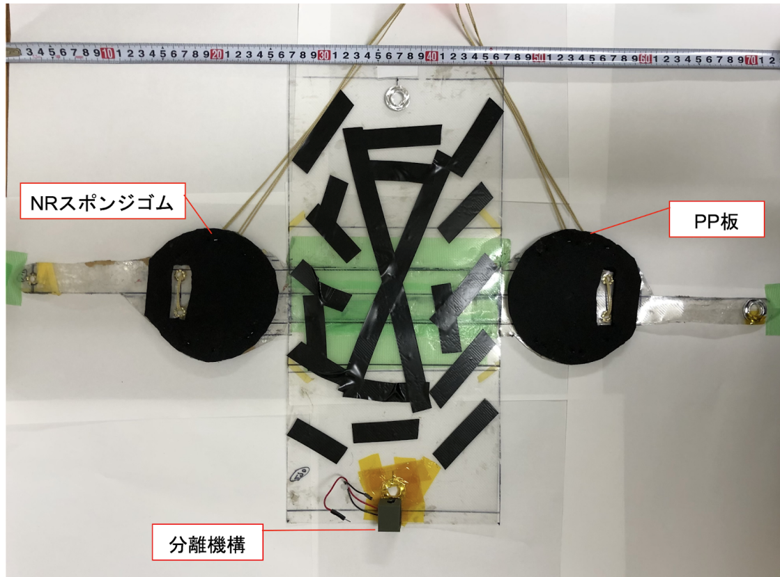
図4.1.9 機体収納用モジュール外観
