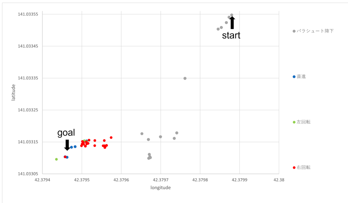
図6.13.3 降下軌跡および走行軌跡
