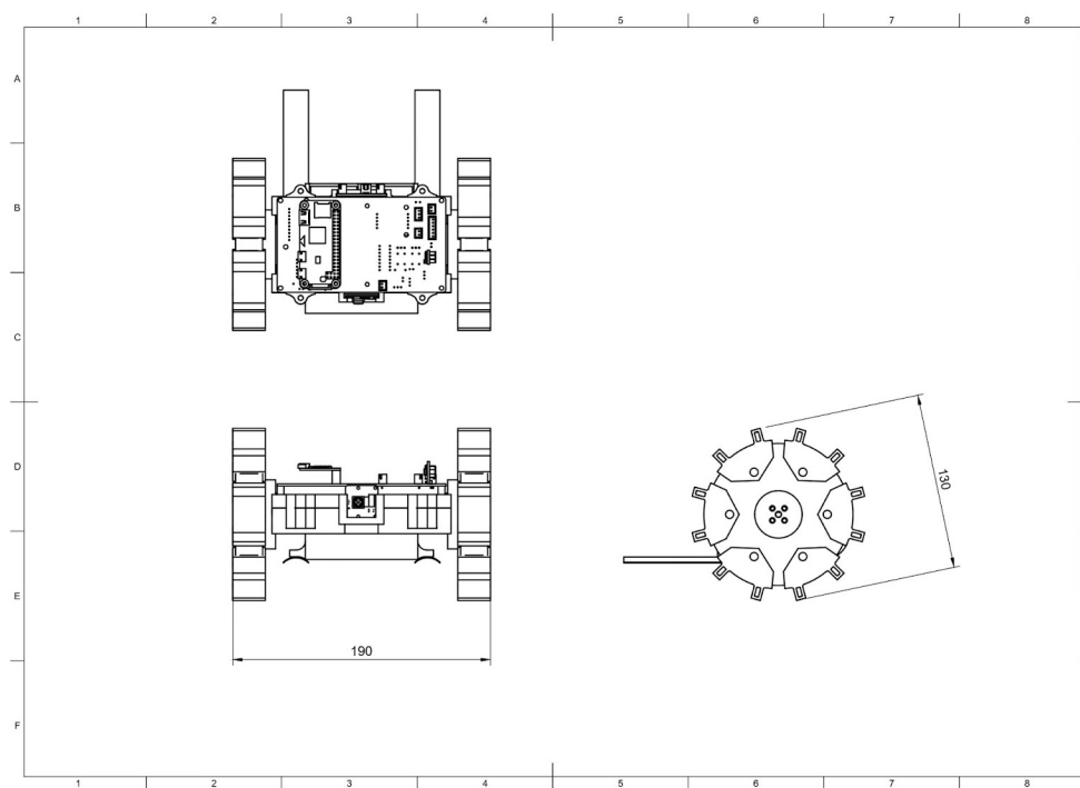
図4.1.4 機体三面図
