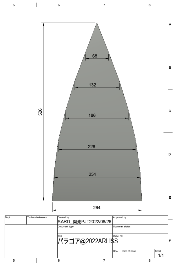
図4.1.8 ゴアの寸法
