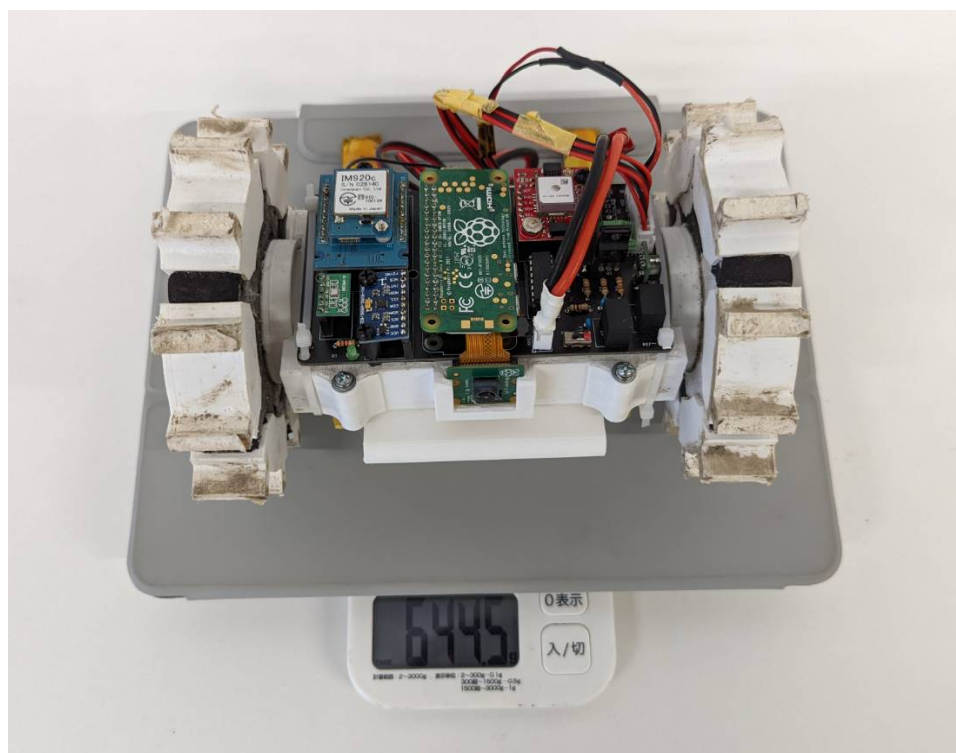
図6.1.1 機体本体の重量（2回目）
