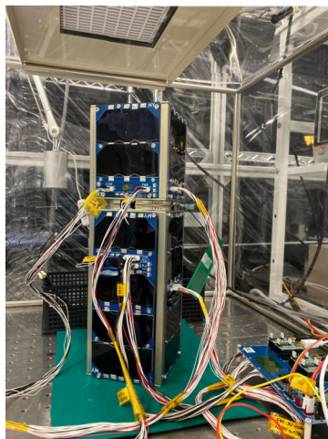
図1 結合時外観
