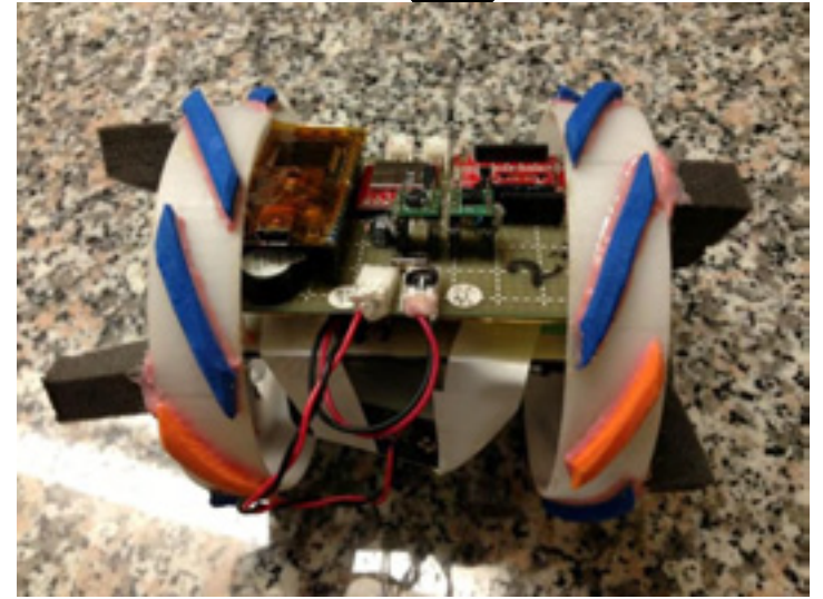
Aoi ローバー Circle size : 105 [mm] Width : 110 [mm] Weight : 413 [g]
